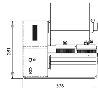
VISTA FRONTALE
