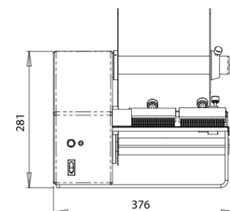
VISTA FRONTALE
