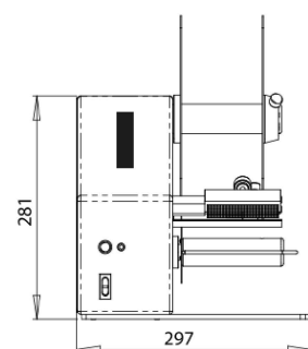
VISTA FRONTALE
