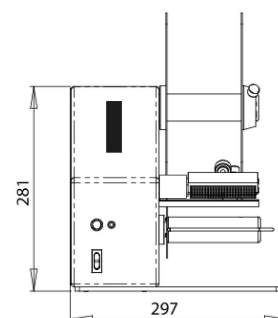
VISTA FRONTALE
