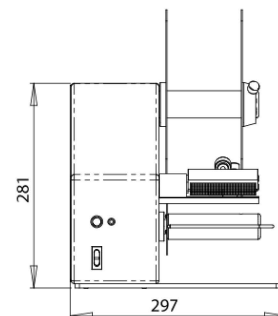
VISTA FRONTALE
